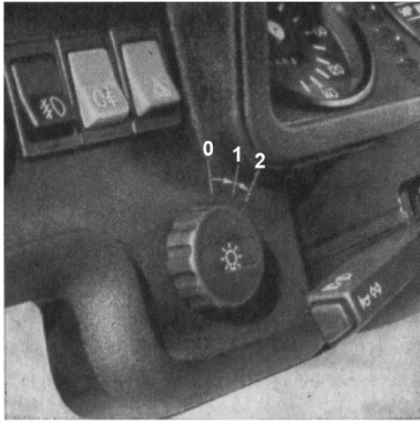
Bild 11: Lichtdreheshalter
