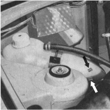
Bild 39: Ausgleichbehälter
